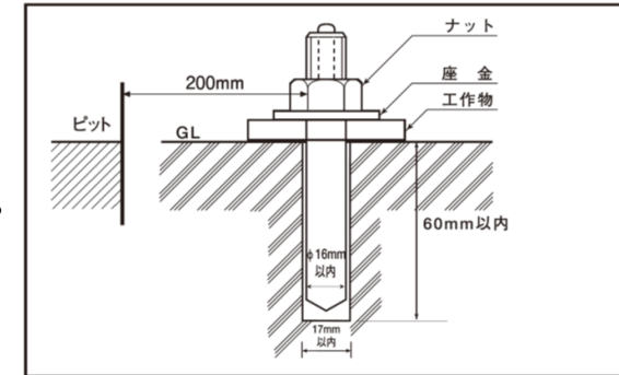
アンカーボルト(オールインアンカー)
